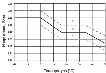
Рис.1. Напряжение заряда в зависимости от температуры при заряде от солнечных панелей.
