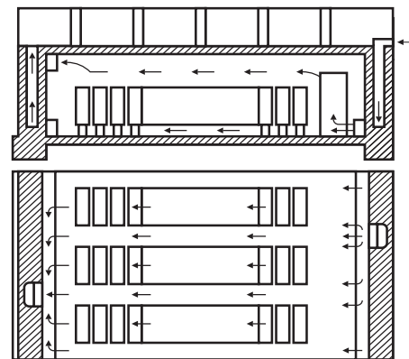
Рис. 4 Организация двусторонней естественной вентиляции.
