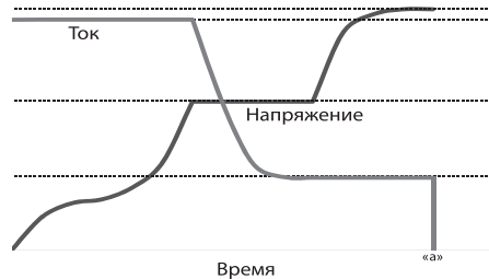
Рис. 3 Зависимость тока и напряжения заряда от времени в режиме IUI, включая фазу заряда малым током и отключение батареи от зарядного устройства (IUIa).
