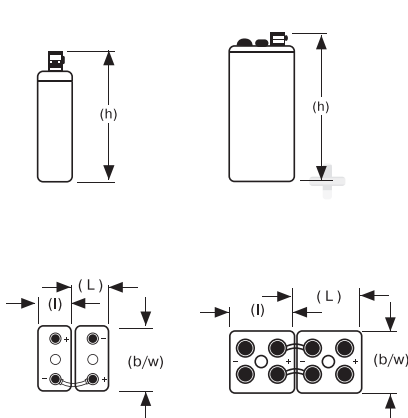
OPzS Solar 190-1080
