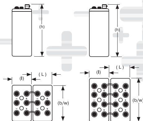
OPzS Solar 3100-3350
