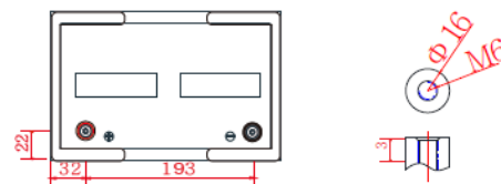
Тип вывода F6
